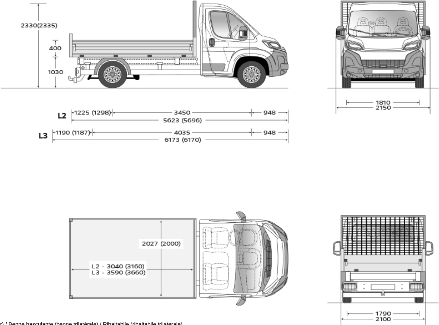
Kipper (Dreiseitenkipper) / Benne basculante (benne trilatérale) / Ribaltabile (ribaltabile trilaterale)
