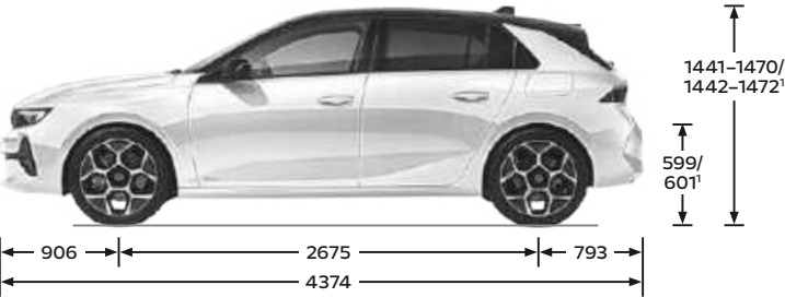
Astra 5 porte Tutte le misure in mm
