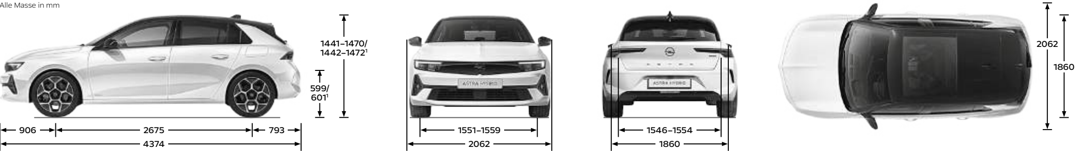
Astra 5-Türer Alle Masse in mm
