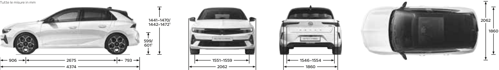
Astra 5 porte Tutte le misure in mm
